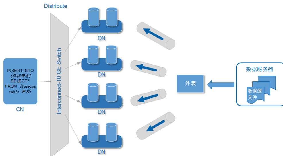
图 3-4 数据并行导入示意图
