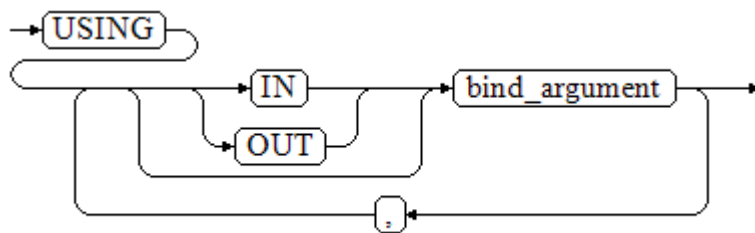
图 11-7 using_clause-1
