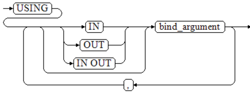
图 11-14 using_clause-4
