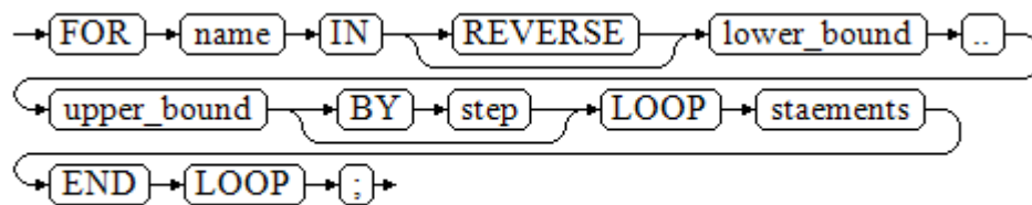
图 11-21 for_loop::=
