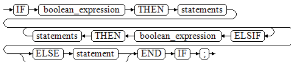
图 11-18 IF_THEN_ELSEIF_ELSE::=
