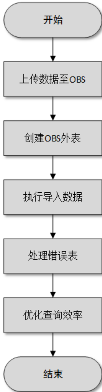
图 3-3 并行导入流程
