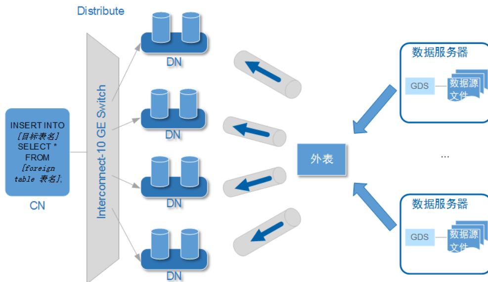
图 3-5 多数据服务器并行导入
