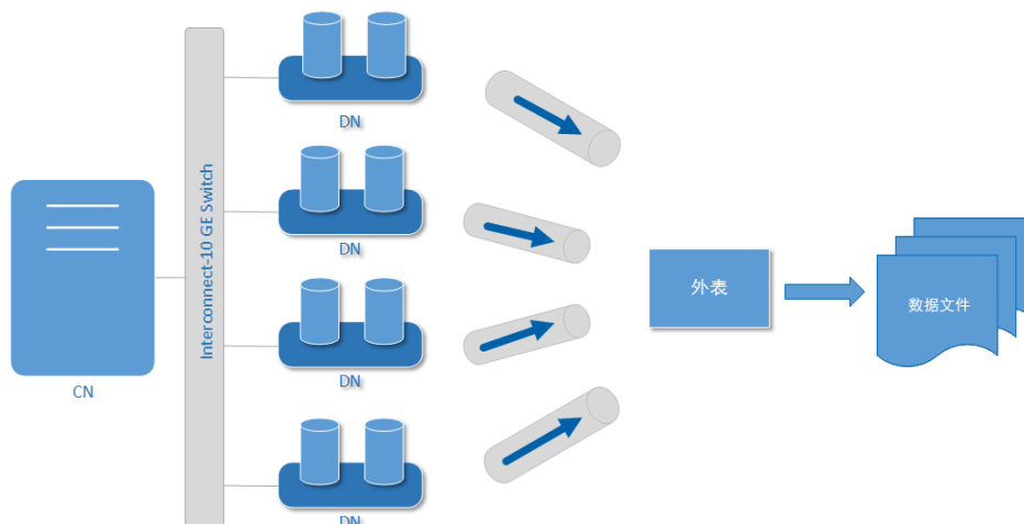
图 3-11 通过外表导出数据
