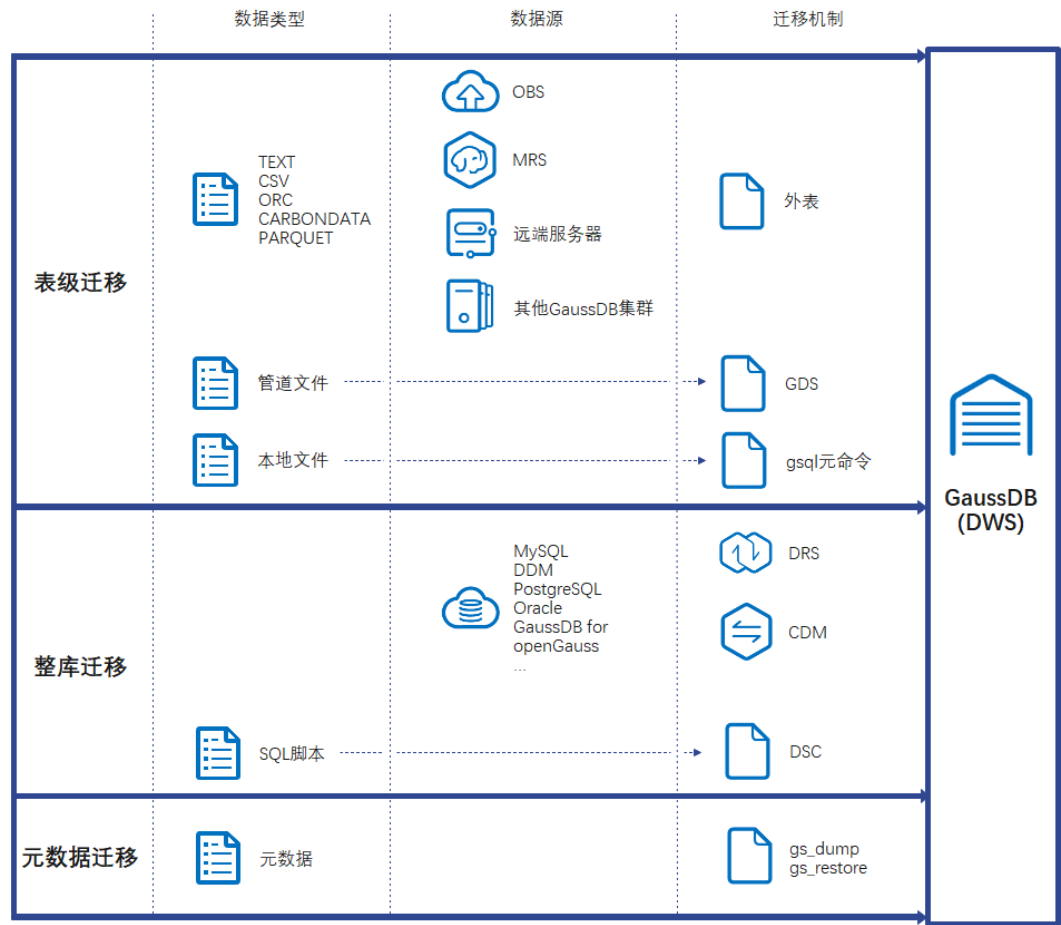
图 3-1 数据迁移示意图
