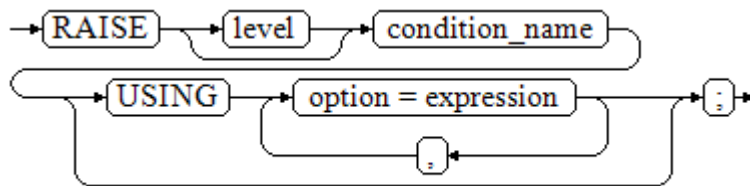
图 11-35 raise_condition::=
