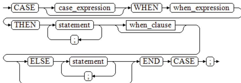
图 11-24 case_when::=
