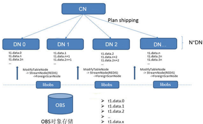
图 3-2 通过 OBS 外表并行导入数据
